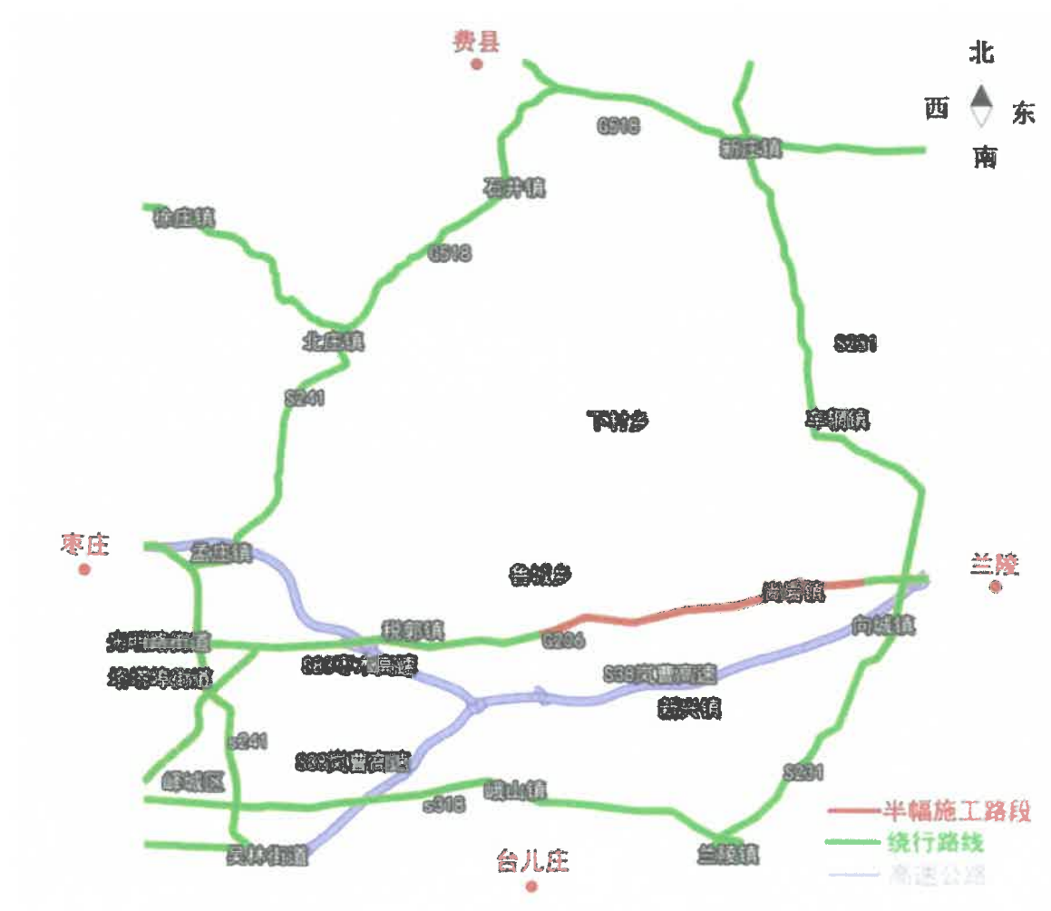
G206威汕线阳明河桥至枣庄界段修复养护工程绕行示意图
